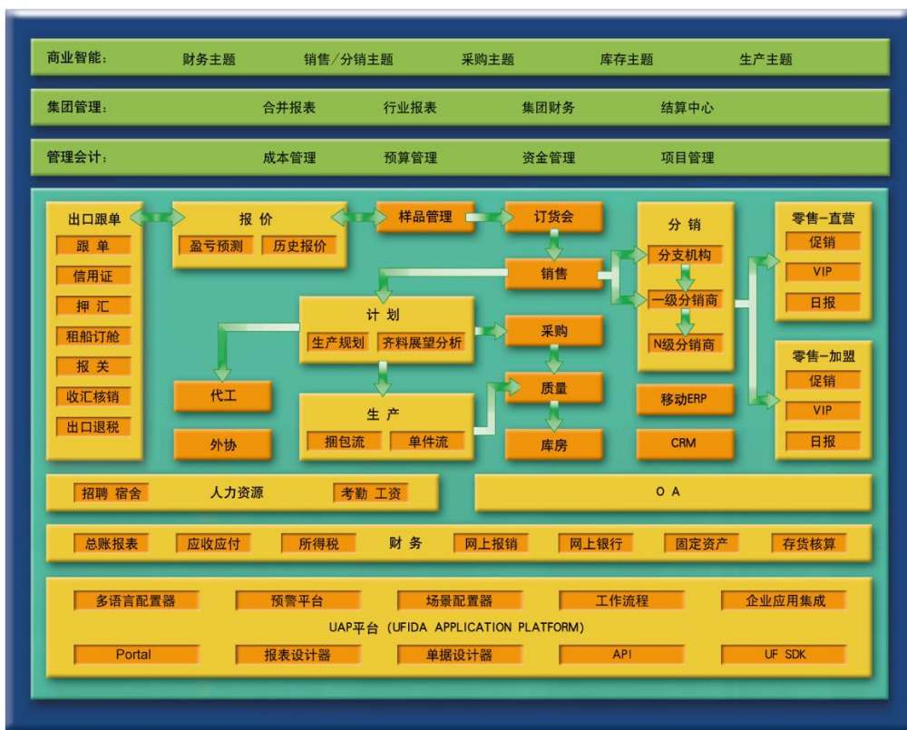
用友 U8 服装行业解决方案关键应用架构图
